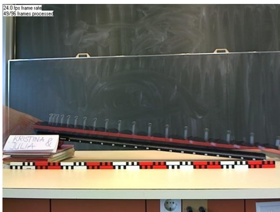
Abb. 8: Von Schülern angefertigtes Bild eines Wagens auf der schiefen Ebene. Für die Auswertung befindet sich ein Meterstab im Bild. Links oben ist die Bildrate eingeblendet.
