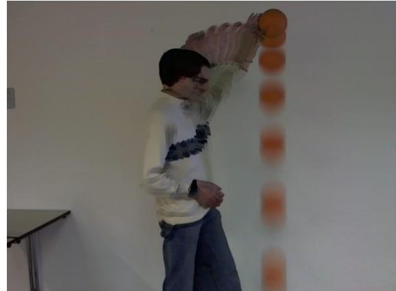
Abb. 5: Fallbewegung einer Kugel
