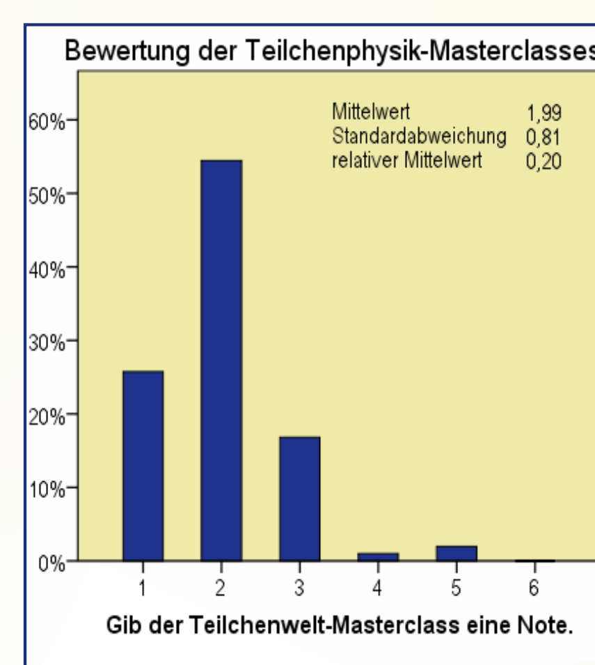
Diagramm 1 - aus der Pilotstudie zu Teilchenphysik-Masterclasses (2011)
