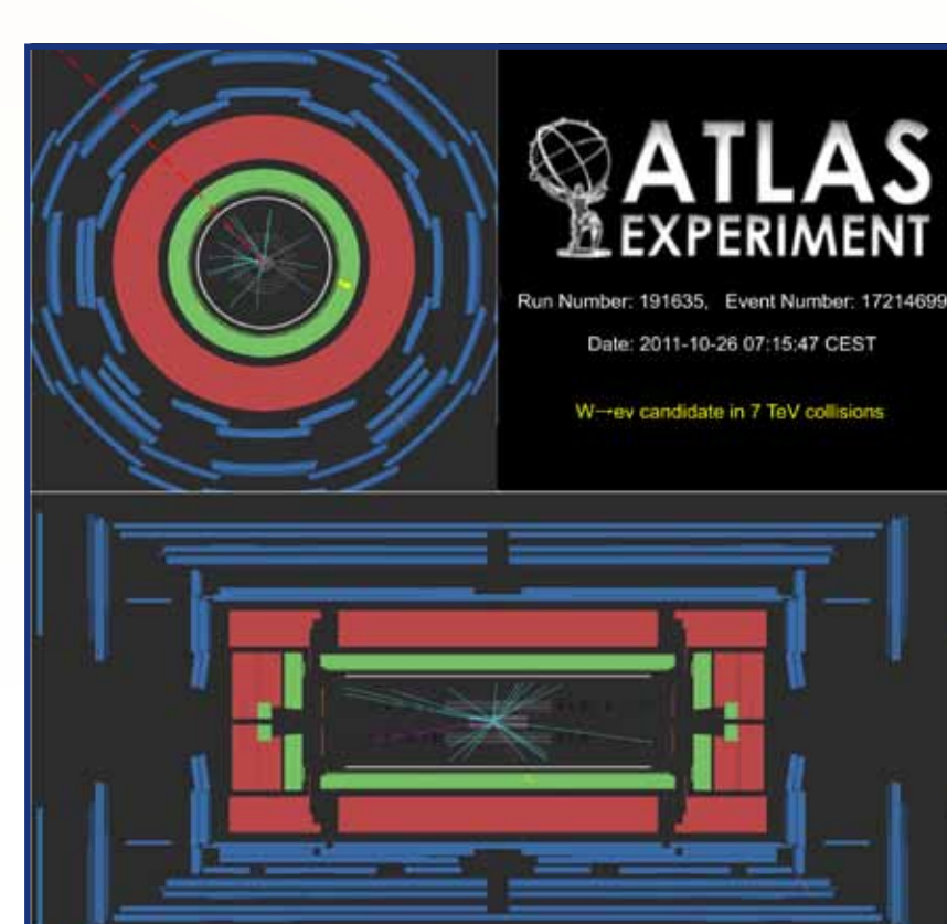
Abb. 3 Durch die Analyse vieler solcher Ereignisse lernen die Teilnehmer die Zusammensetzung des Protons kennen.
