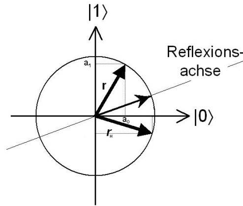
Abb.2: Graphische Veranschaulichung der Hadamard-Transformation
