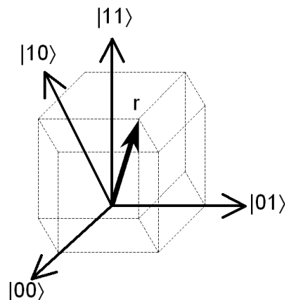
Abb.1: Zustandsvektor r eines aus zwei Quantenbits aufgebauten Quantenregisters.
