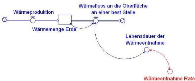
Abb. 9: Bei der lokalen Geothermie ist die Lebensdauer der Wärmeentnahme abhängig von der Wärmeentnahmerate. Wenn die Geothermie-Anlage nachhaltig geführt wird, handelt es sich um eine erneuerbare Energiequelle, ansonsten um eine nicht erneuerbare Energiequelle.
