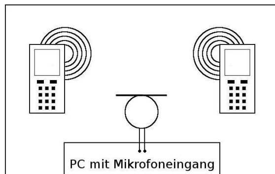
Abb. 7: Versuchsaufbau zur Erzeugung einer akustischen Schwebung; wenn der PC nicht über ein eingebautes Mikrophon verfügt, so kann auch ein Headset oder ein weiteres Handy zum Einsatz kommen.
