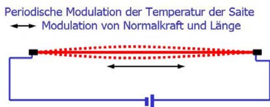
Abb.3: Die so hervorgerufenen Temperaturos zillationen bewirken eine Modulation der thermischen Ausdehnung, in deren Folge auch die Normalkraft variiert, mit der die Saite eingespannt wird (angedeutet durch den schwarzen Pfeil).
