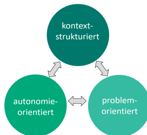
Abb. 1: Angezielte Schülerlabor-Charakteristika
