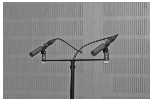
Abb. 6: Mikrofonanordnung für die Laufzeitstereophonie.
