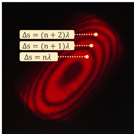
Abb.3: Interferenzmuster
